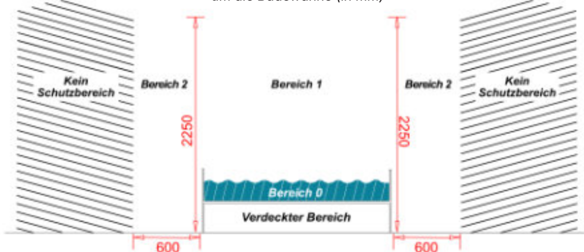
Elektrische Schutzbereiche rund um die Badewanne (in mm)
